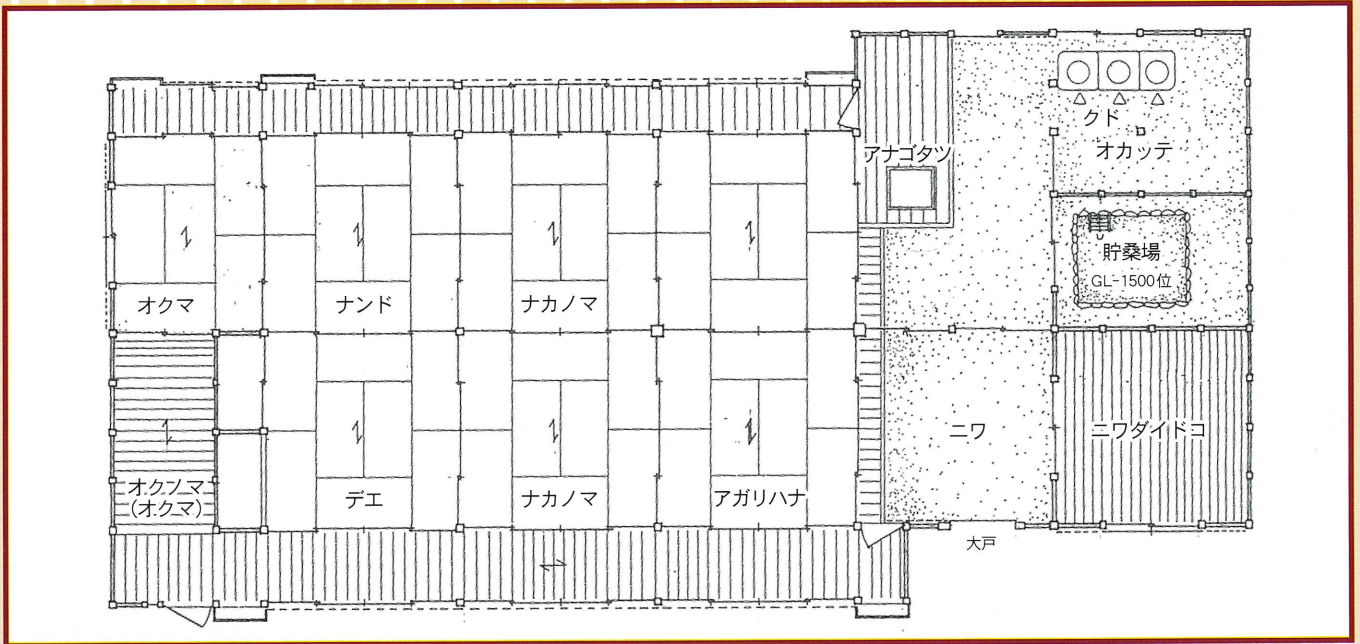
養蚕民家の復元平面図
