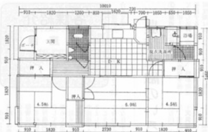
B'-16 (西入口) 平面图 53.0m 2 (16坪)
