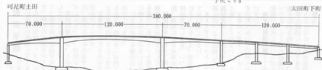
中濃大橋完成予想図
