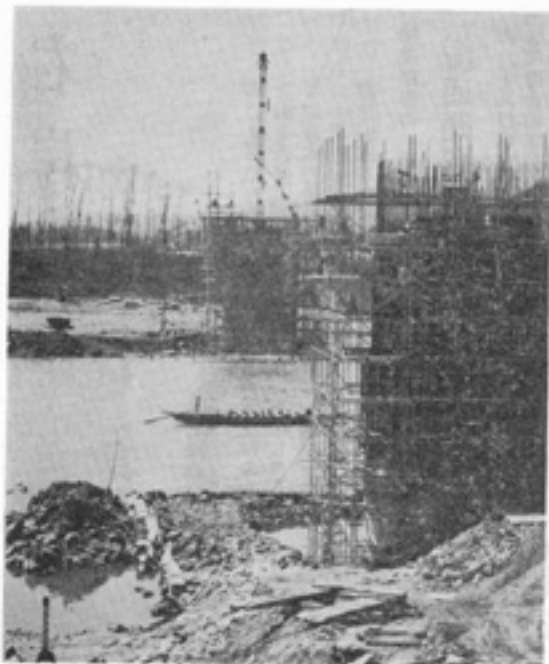
美濃加茂市と可児町を結ぶ中濃大橋の架橋工事は、4月に入って橋台工事が始まりました。
