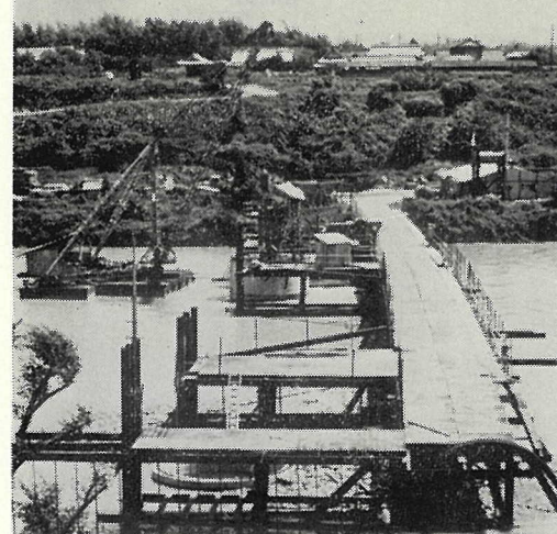
橋脚工事が進む川合大橋
