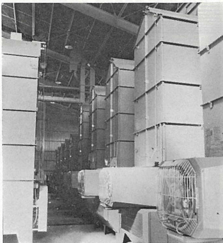
1万俵が処理できる粃すり機
