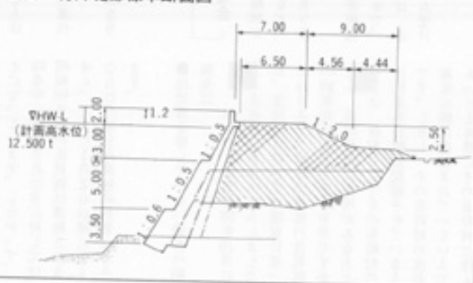
図(2) 特殊堤部標準断面図
