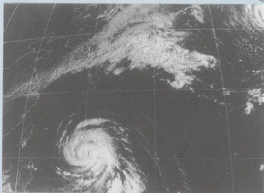
9. 28災害で大雨をもたらした台風10号
