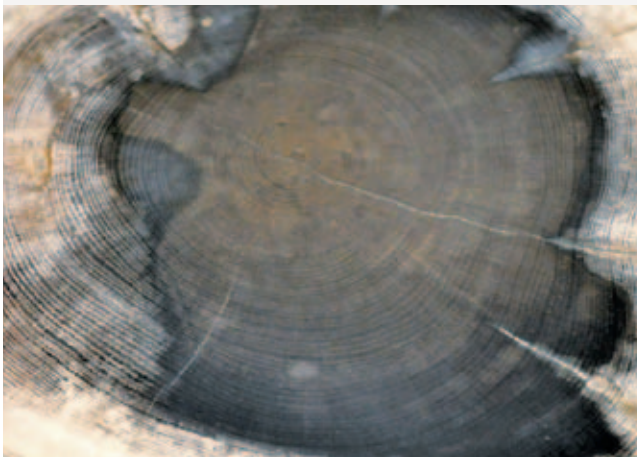
「珪化木の年輪」
